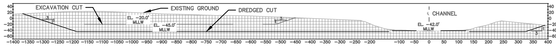
B1 SECTION AT LNG PLATFORM W-0006
